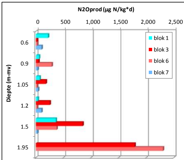
Figuur 141 Verloop potentiële denitrificatie met het bodemprofiel.
