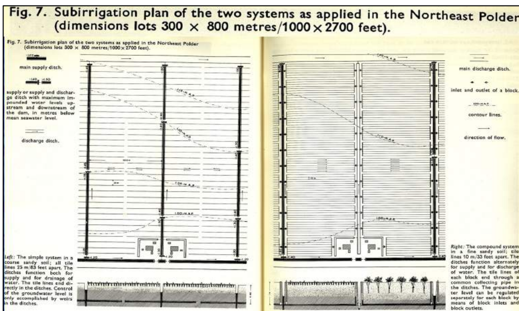
Figuur 23 Twee systemen voor sub-irrigatie in de Noordoostpolder: het enkelvoudige systeem, waarin drainbuizen in sloten uitmondten (links) en het samengestelde systeem waarin de drains waren aangesloten op verzameldrains (rechts).
