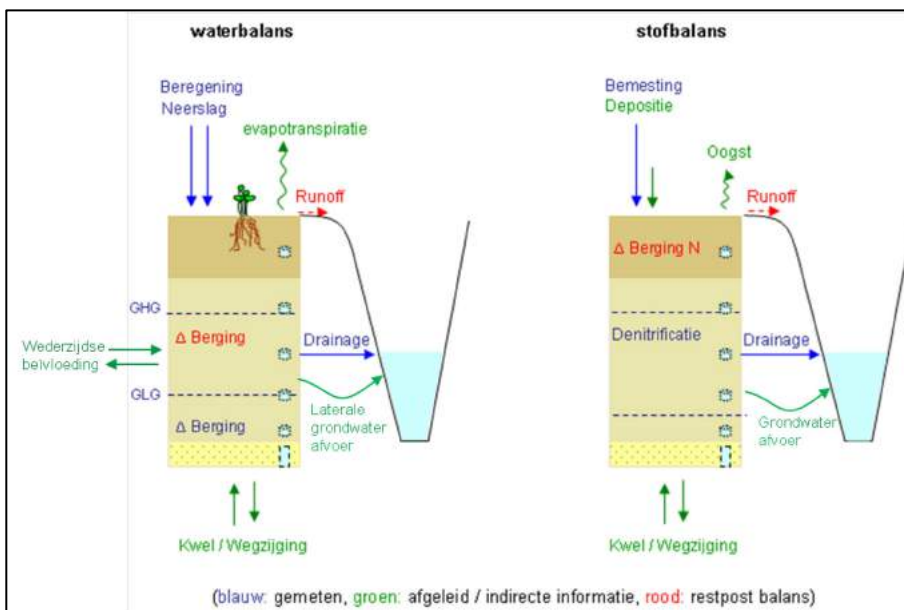
Figuur 148 Schematische weergave van de water- en stoffenbalans op 'Rusthoeve'.
