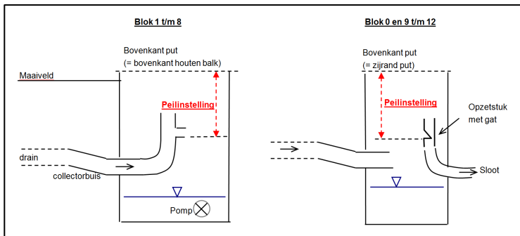
Figuur 147 Peilinstellingen in regelputten (links) en bufferputten op proeflocatie 'Rusthoeve'.
