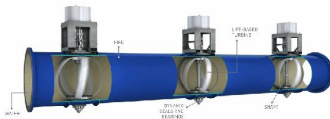
Afbeelding 3.5 Restdrukturbines op het waterleidingnet
