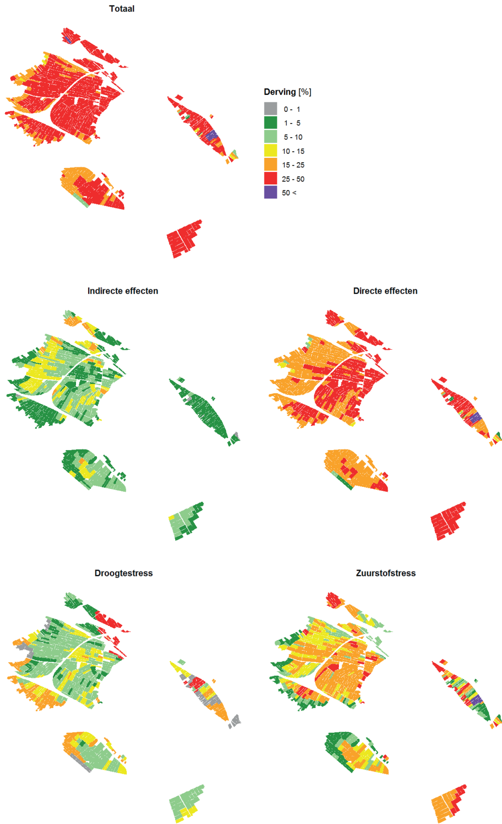
FIGUUR 3.4 LANGJARIG GEMIDDELTE OPBRENGSTDERVING IN NAARDERMEER [%] MET BOVEN DE TOTALE OPBRENGSTDERVING, MIDDEN UITSPLITSING NAAR INDIRECTE EN DIRECTE EFFECTEN EN ONDER UITSPLITSING NAAR DROOGTESTRESS EN ZUURSTOFSTRESS
