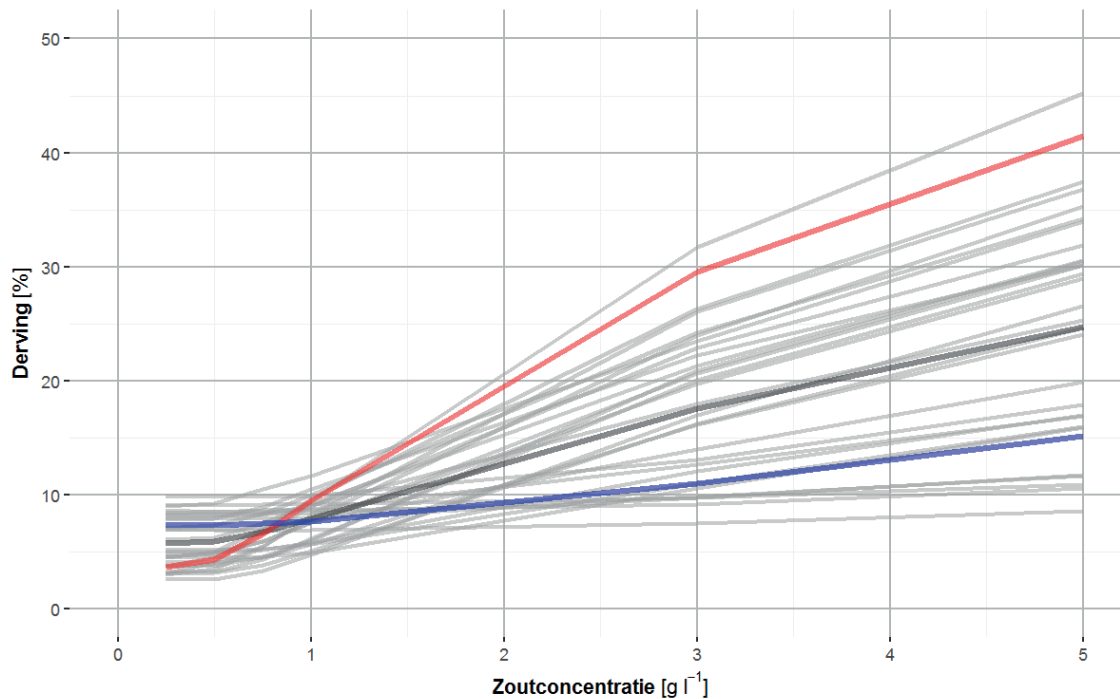
FIGUUR 4.4 GEMIDDELDE OPBRENGSTDERIVING VOOR DE HAARLEMMEERPOLDER BIJ OPLOPENDE ZOUTCONCENTRATIE IN HET BEREGENINGSWATER VOOR CONSUMPTIEAARDAPPELEN VOOR DE PERIODE 1981 – 2010 [%], MET IN HET DONKERGRIJS DE LANGJARIG GEMIDDELDE OPBRENGSTDERIVING EN IN ROOD EN BLAUW DE OPBRENGSTDERIVING VOOR RESPECTIEVELIJK EEN DROOG JAAR (2003) EN EEN NAT JAAR (1998)
